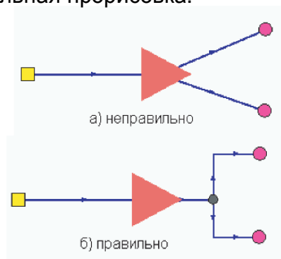
Рисунок 7.9 - Отображение ЦТП
